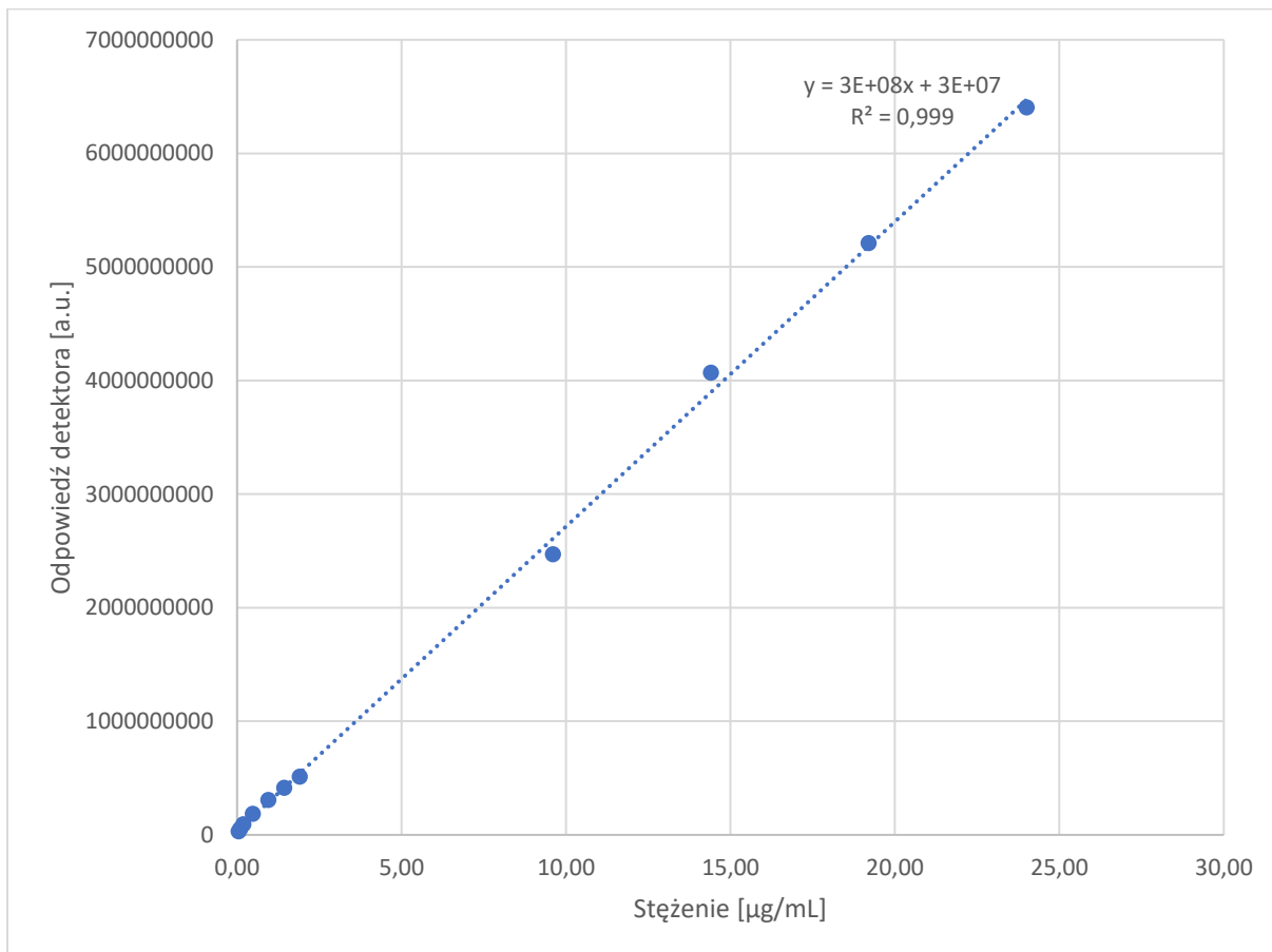
Rys. 1. Wykres kalibracyjny dla Kordycepiny uzyskany za pomocą LC-HRMS.
